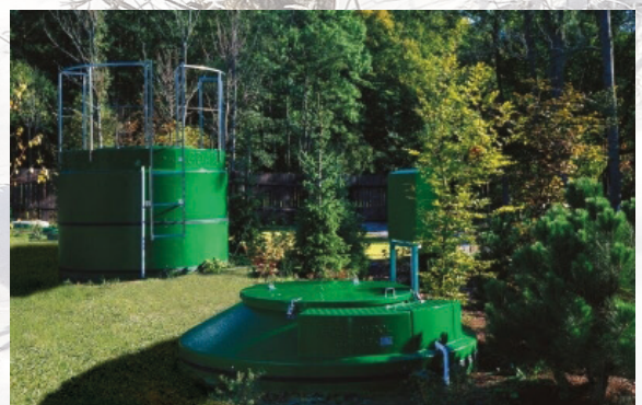
Budowa oczyszczalni w Zdrzewie wraz z siecią kanalizacyjną
